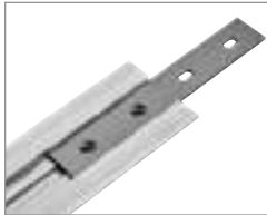
Carril (parte inferior) con la unión de carril parcialmente instalada
